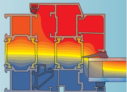
Sisään avattava ikkuna Inward opening window
