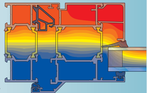
Ulos avattava ikkuna Outward opening window
